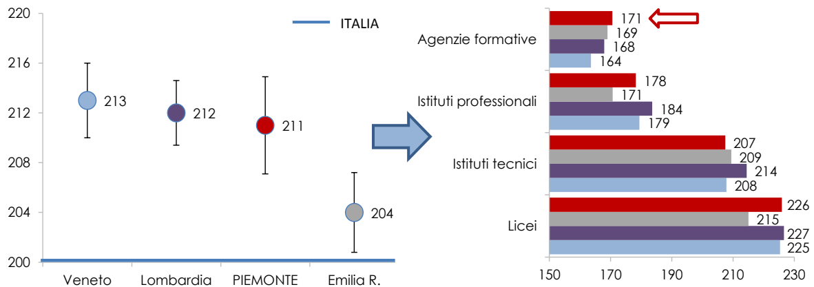
Fig. 3.10 Risultati in matematica in Piemonte, Lombardia, Veneto e Emilia Romagna, Il ciclo, 2016
